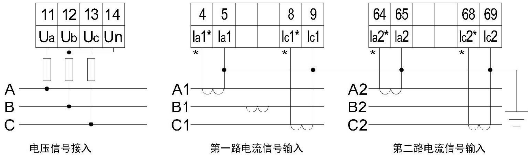
三相三线接线
