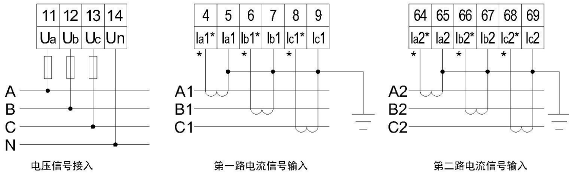
三相四线接线
