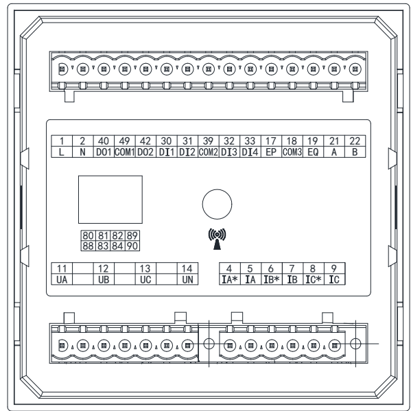
图 18 APM520 扩展 WF/LoRa 接线图
