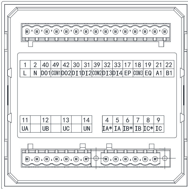
图 13 APM520 基础款接线图
