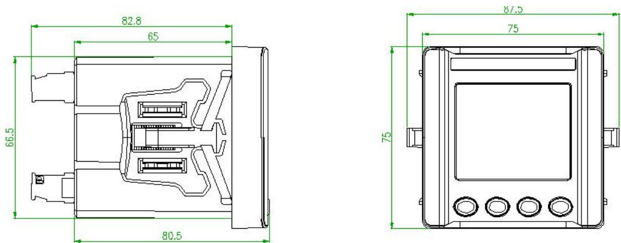
图 2 APM510 尺寸图
